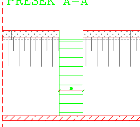
PRESEK A-A
