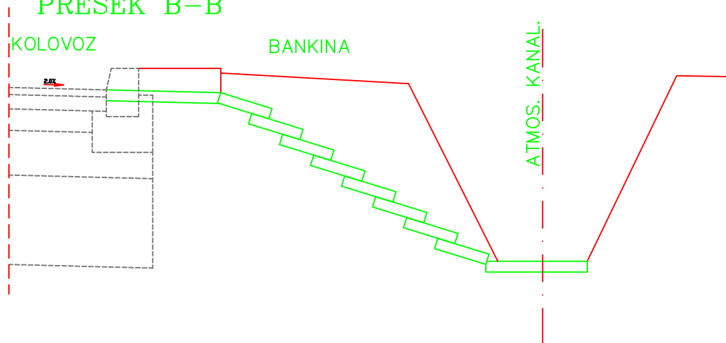
PRESEK B-B
