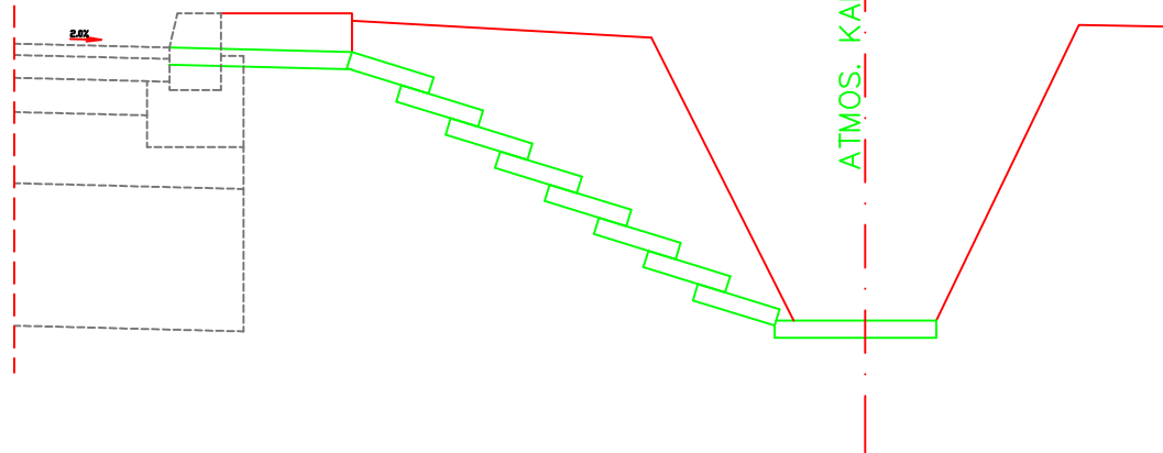
PRESEK B-B
