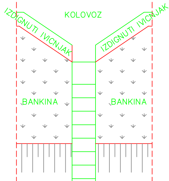
IZGLED ODOZGO
