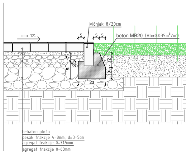
Detalj ivičnjaka I3 (8/20) do zelenila -beton u ravni zelenila-
