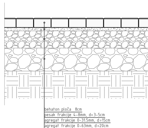
DETALJ TAMPON SLOJEVA NA FLEKSIBILNOJ KONSTRUKCIJI U delu staze kuda prolazi vozíč
